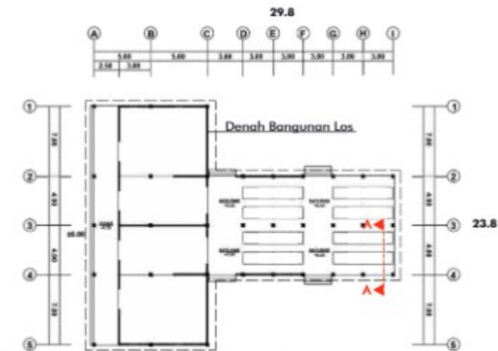
Dimensi bangunan Los sumber: Dokumentasi pribadi (2020)
