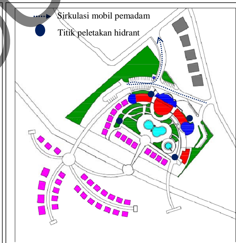
KONSEP SISITIM PEMADAM KEBAKARAN
