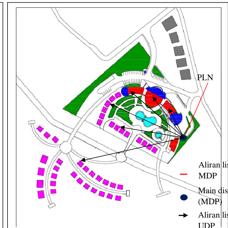
KONSEP SISITIM JARINGAN LISTRIK
