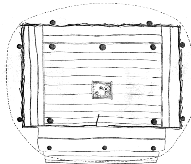
Denah rumah adat Maubisse sumber : Arqitectura timorensse
